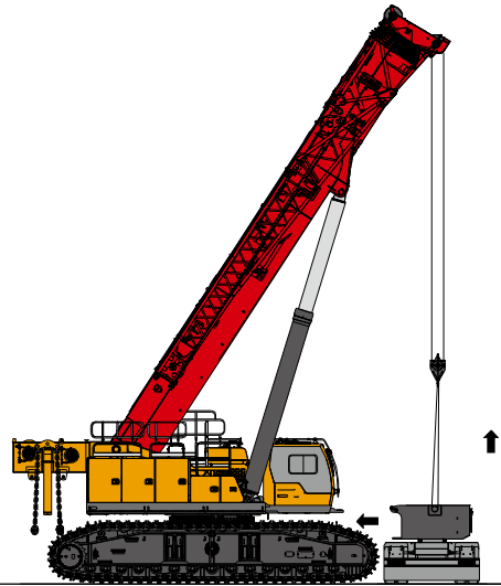
7 Carbody CW installation 中央配重安装
