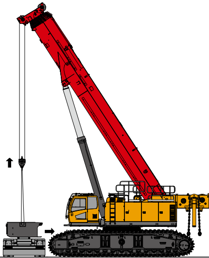
6 Carbody CW installation 中央配重安装
